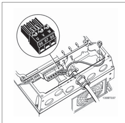
Рисунок 5.9: Подключение двигателя в случае корпуса A5
