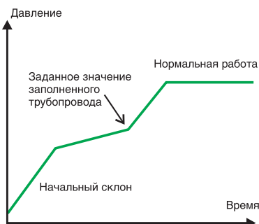
Режим заполнения трубопровода для предотвращения гидравлического удара
